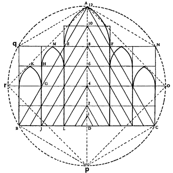
Disegno di Gabriele Scovaloca per la progettazione dell'alzato del Duomo di Milano (1392)
