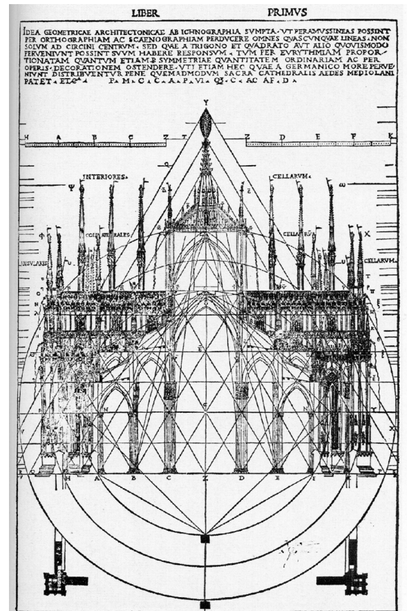
Sezione trasversale del Duomo di Milano
